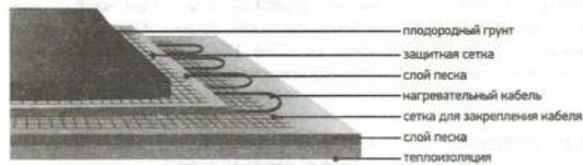
Рисунок 3. Схема укладки в разрезе.
