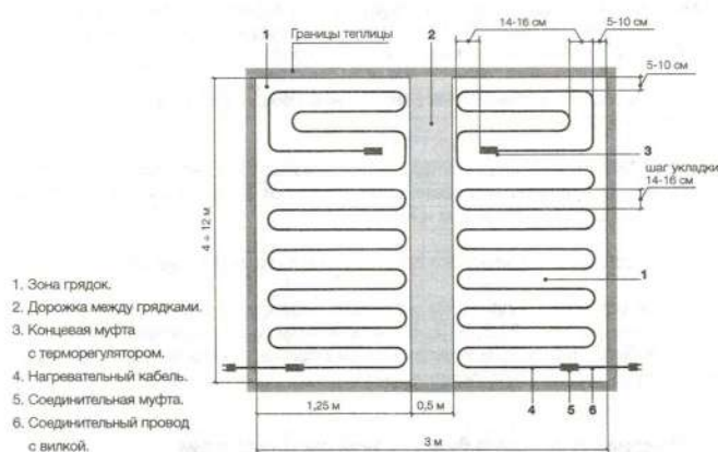
Рисунок 2. Схема укладки нагревательной секции для обогрева грунта теплицы.
